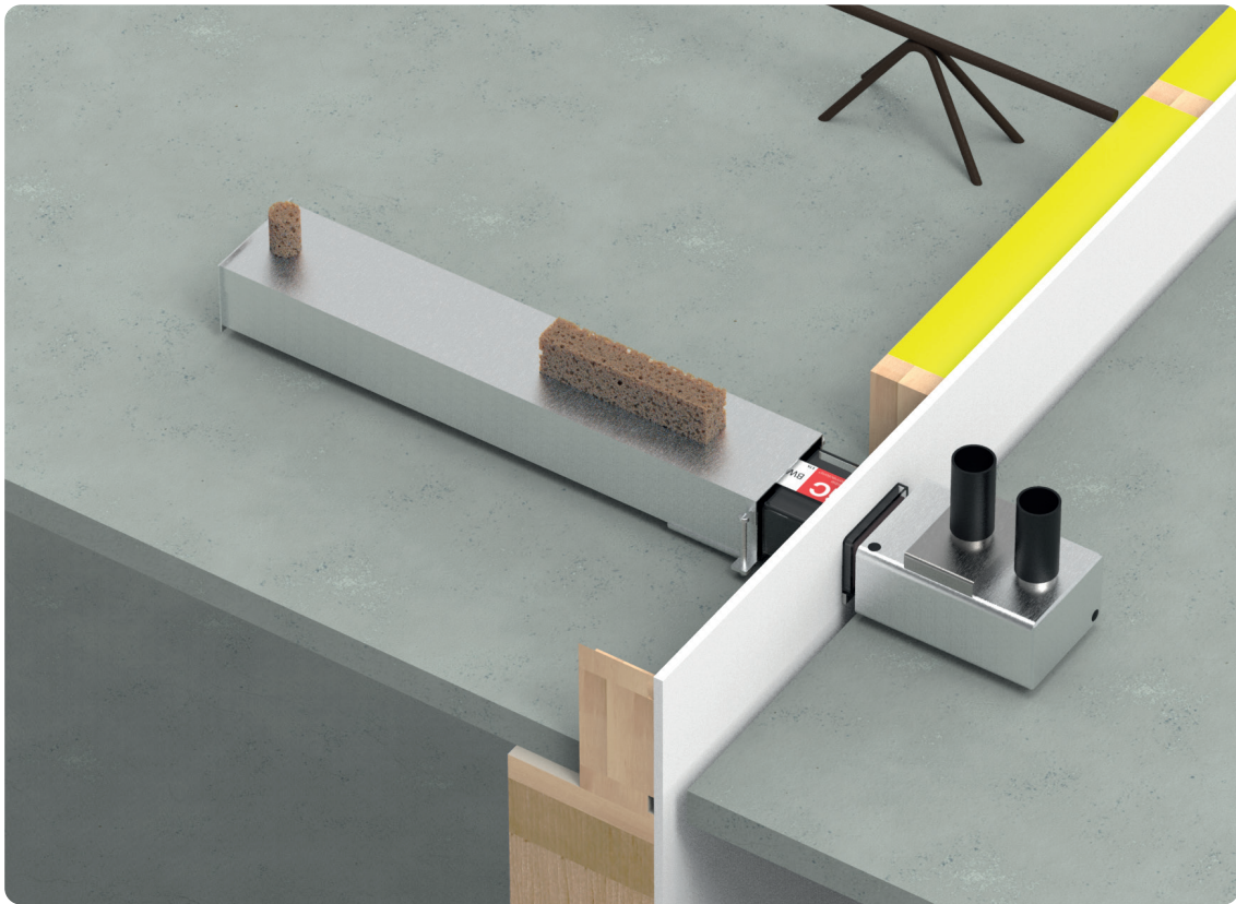
Modell av BWC 55-light med BWC-4 (balkongboks). Se modellen under for armeringseksempel
