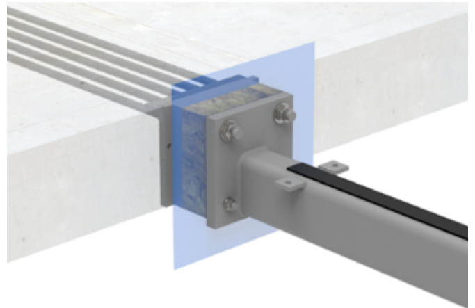
BWC U-H innstøpt og montert til betongdekke.
