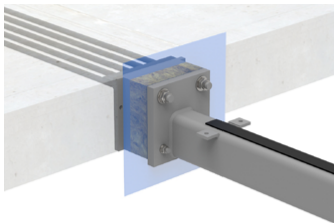
BWC U-H innstøpt og montert til betongdekke.
