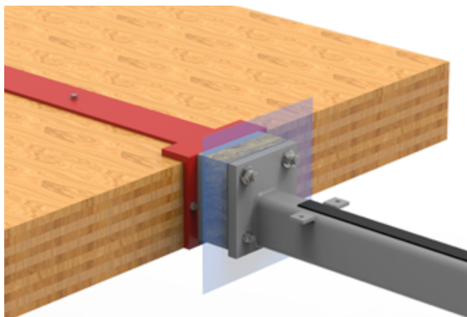
BWC U-H montert til massivt tredekke.
