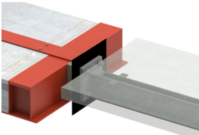
BWC U-H montert på HSQ bjelke.
