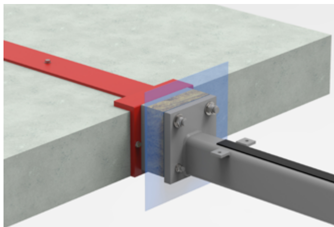
Rehabilitering av bolig, ettermontering av utkragede balkonger på etablerte/eksisterende/transformerte bygg.
