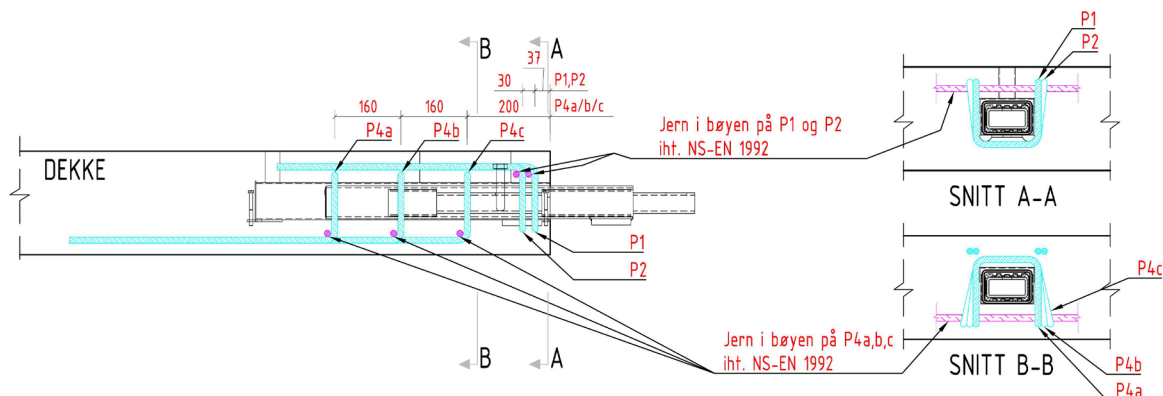
Figur 1: Utforming forankringsarmering – Eksempel A. Denne utformingen kan ofte være passende når enheten ligger på langs av dekkets spennretning.
