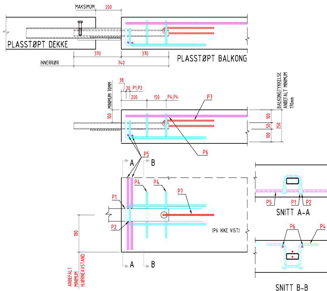
Figur 4: Eksempel - Forankringsarmering i balkong. Ved bruk av innerrør uttrekt 370mm.
