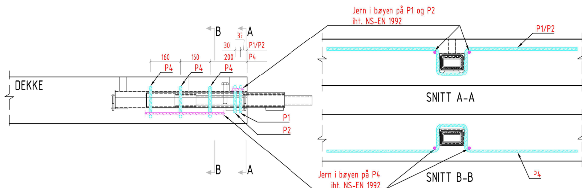
Figur 2: Utforming forankringsarmering – Eksempel B. Denne utformingen kan ofte være passende når enheten ligger på tvers av dekkets spennretning.
