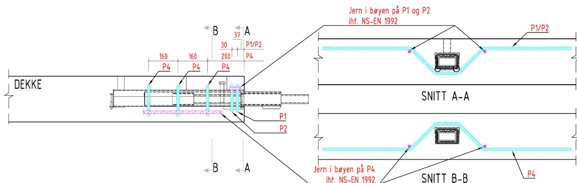
Figur 3: Utforming forankringsarmering – Eksempel C.
