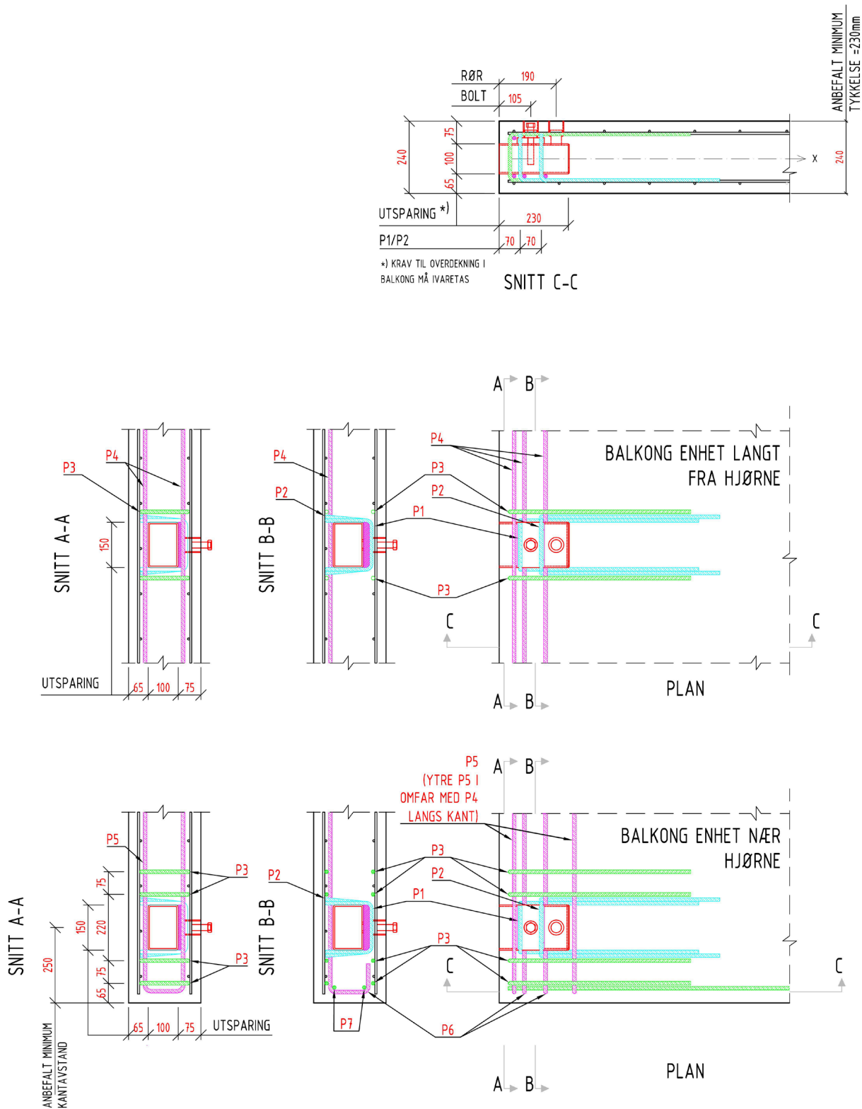
Figur 5: Forankringsarmering i balkong. Ved bruk av balkongboks.
