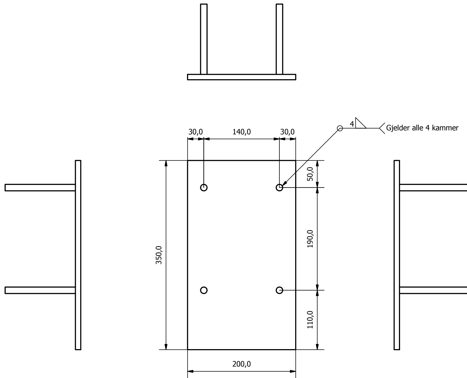
Målestokk 1:4
